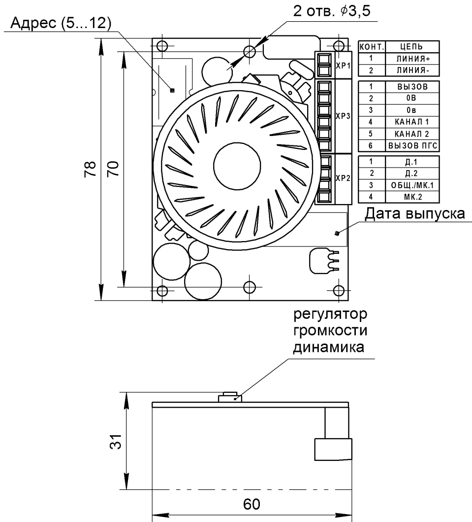
Рис.1 Внешний вид Устройства переговорного УП-МД НШЕК.465112.010
